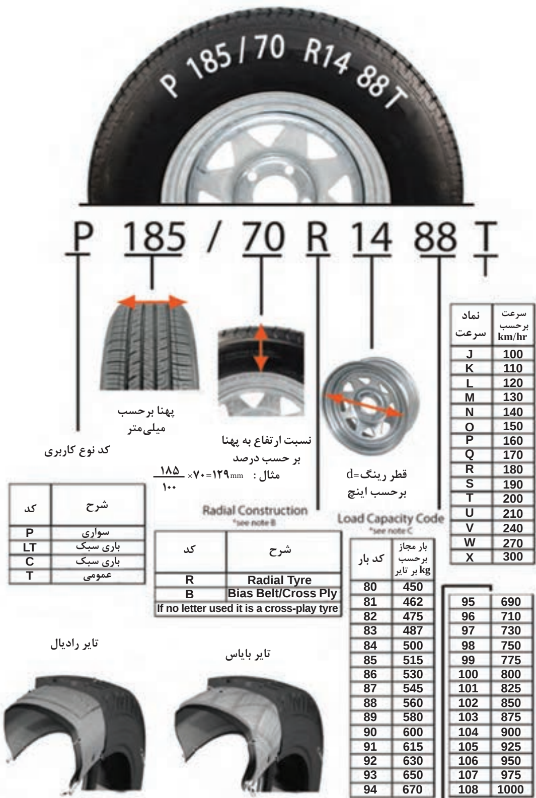
شکل ۷- مفهوم کدهای اصلی درج شده روی تایر
