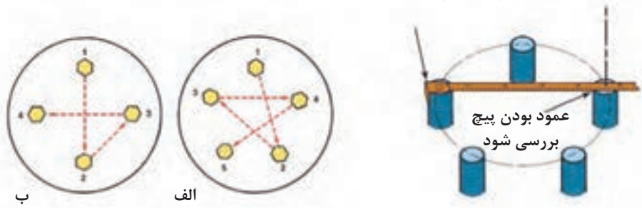
شکل ۲۰- روش صحیح بستن پیچ یا مهره چرخ و کنترل ارتفاع پیچ
