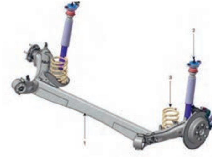
شکل ۴۷- مرکب پیچشی
