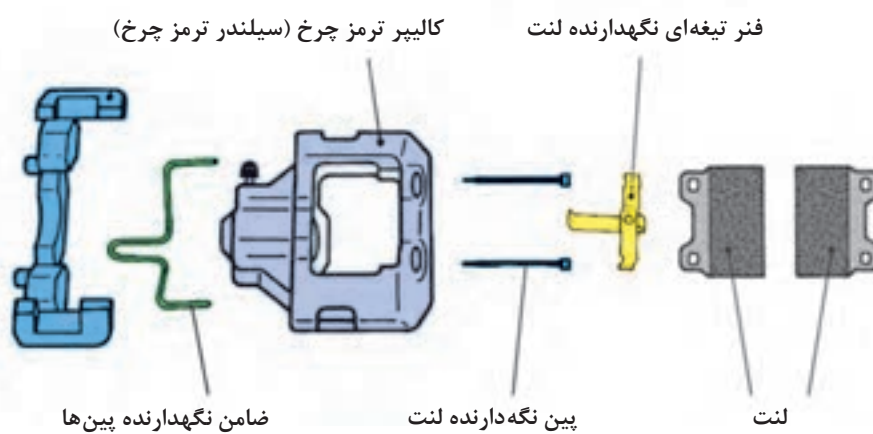
شکل ۱۰- سیستم ترمز دیسکی
