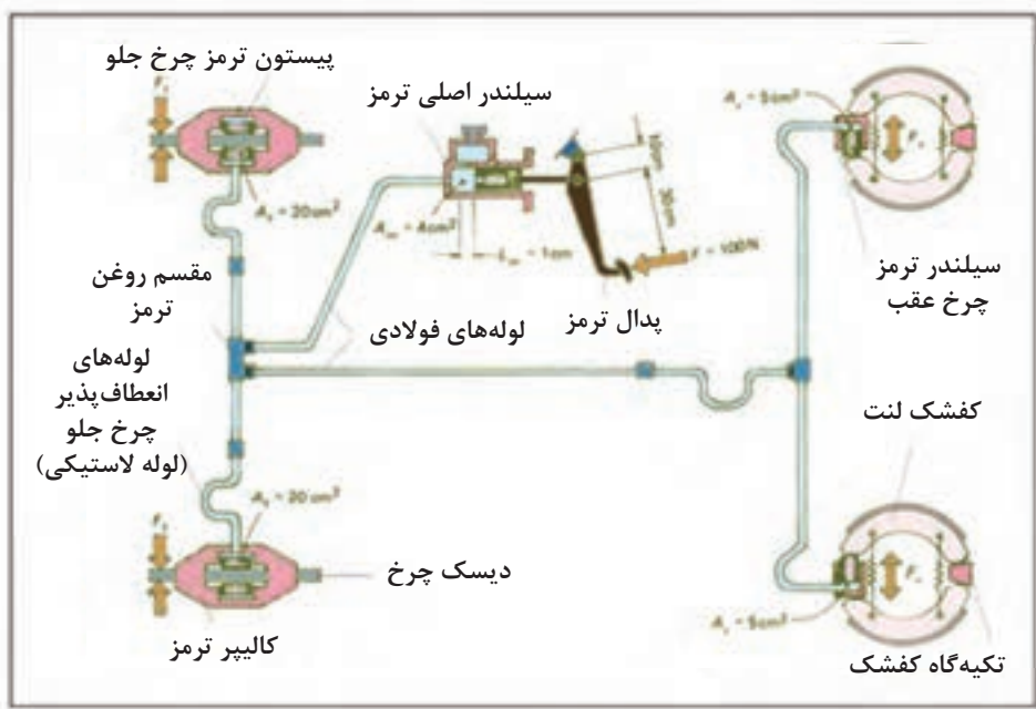
شکل ۲- شماتیک سیستم ترمز هیدرولیکی تک مداری
